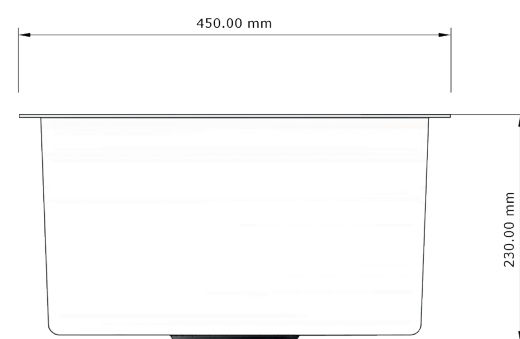
VISTA LATERAL
