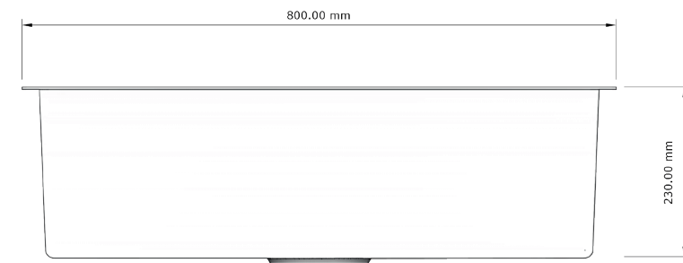
VISTA FROTAL
